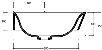
Sezione A-A Section A-A
